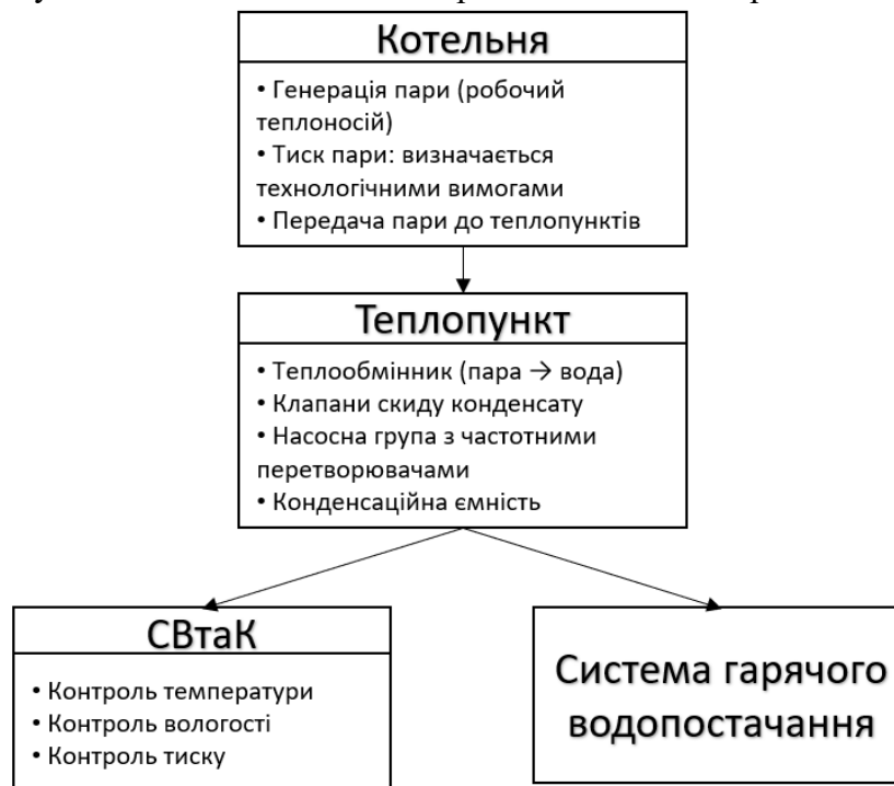
Рисунок 1 – схема теплоенергетичного господарства
