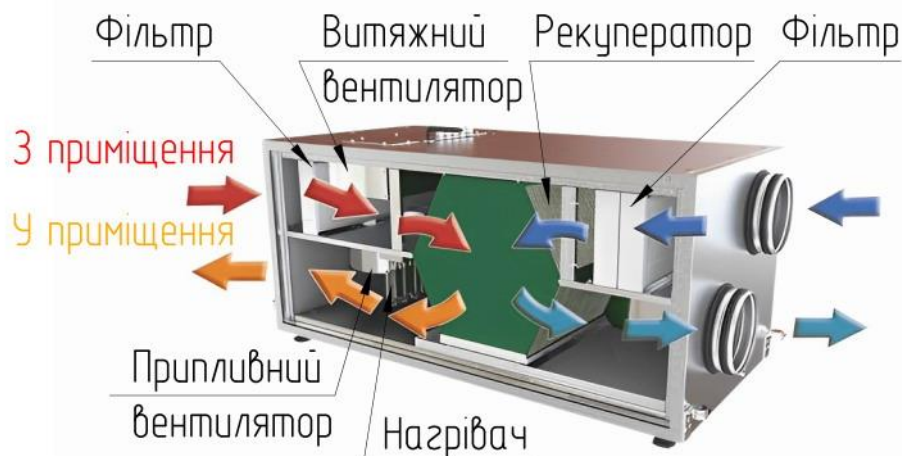
Рисунок 2 – Типова схема вентиляції з рекуперацією тепла [5]
