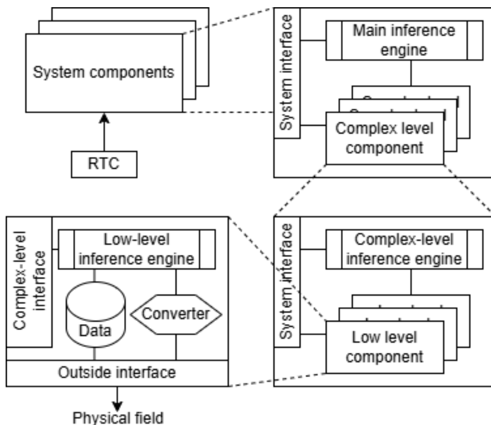
Рисунок 1 – Ієрархічна структура об'єкту
