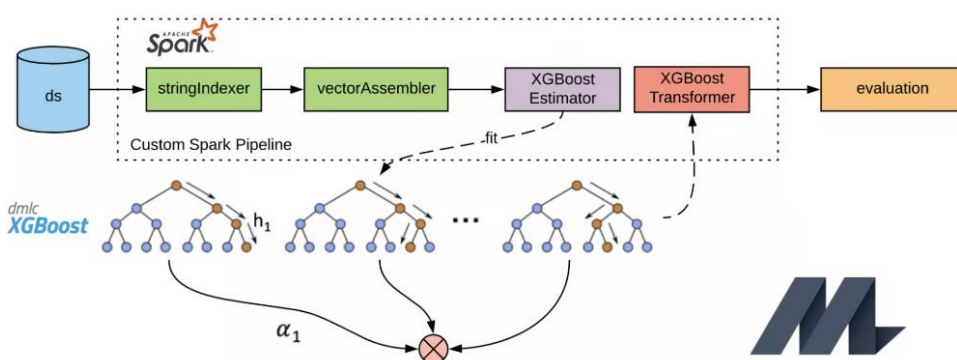
Рисунок 2 – XGBoost для навчання моделей глибокого дерева
